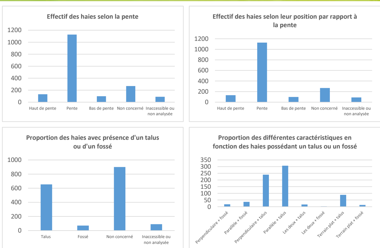
Figure 4 : Analyse de la fonction hydrologique des haies
